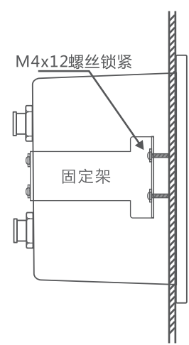
图3 嵌入式安装 (开孔尺寸: 151 X 102mm)
