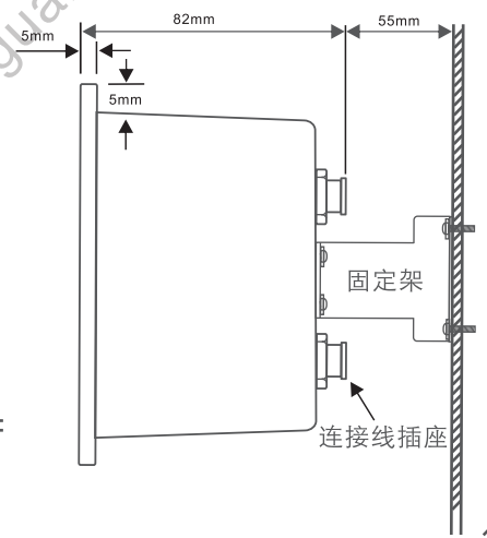
图2 壁挂式安装
